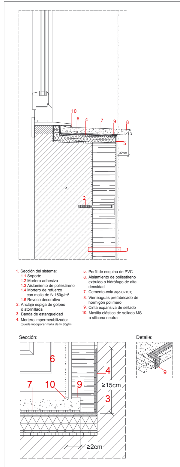
Detalle de alféizar de ventana. Sección vertical. Vierteaguas prefabricado de hormigón. Acabado con revoco.
