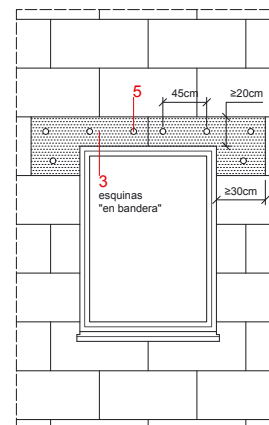
Detalle de cortafuegos. Sección vertical. Barrera de lana de roca en dintel de ventana. Acabado con revoco.
