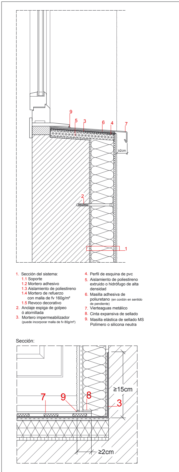
Detalle de alféizar de ventana. Sección vertical. Vierteaguas metálico. Acabado con revoco.
