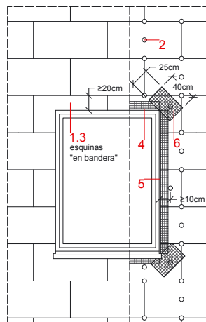
Detalle de dintel de ventana. Sección vertical. Encuentro con carpintería. Acabado con revoco.
