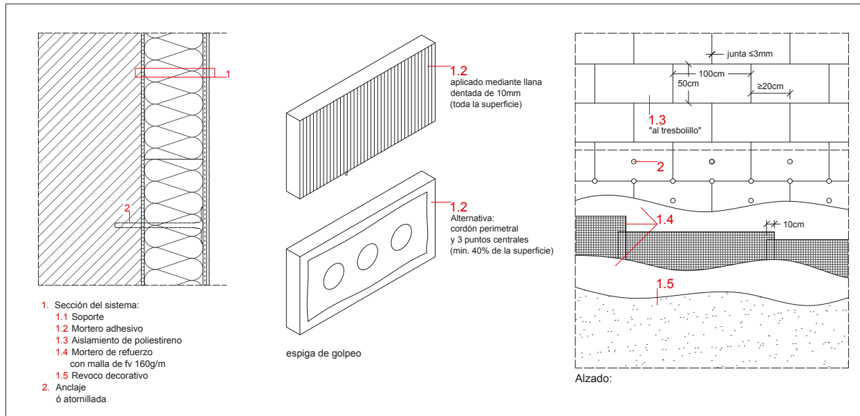
Detalle del sistema. Sección vertical. Adhesión de paneles. Acabado con revoco.
