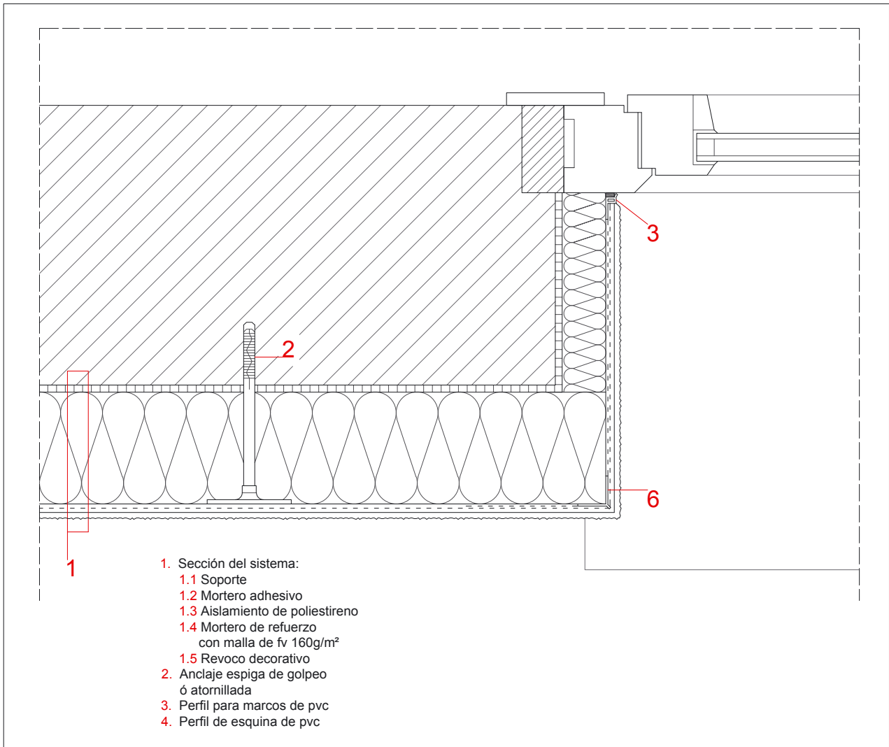
Detalle de mocheta de ventana. Sección horizontal. Encuentro con carpintería. Acabado con revoco.
