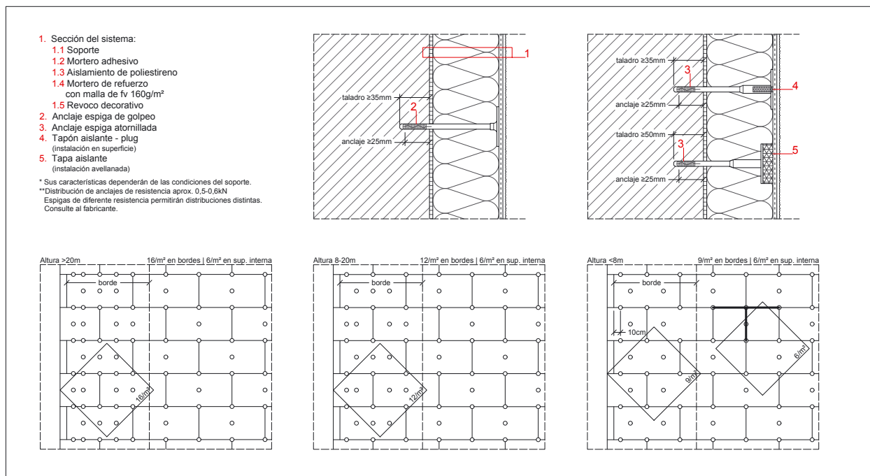
Detalle de espigas. Sección vertical. Instalación* y distribución de fijaciones en función de la altura**. Acabado con revoco.
